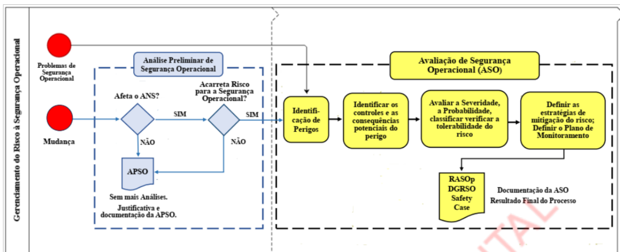
Fluxograma Gerenciamento de Risco
